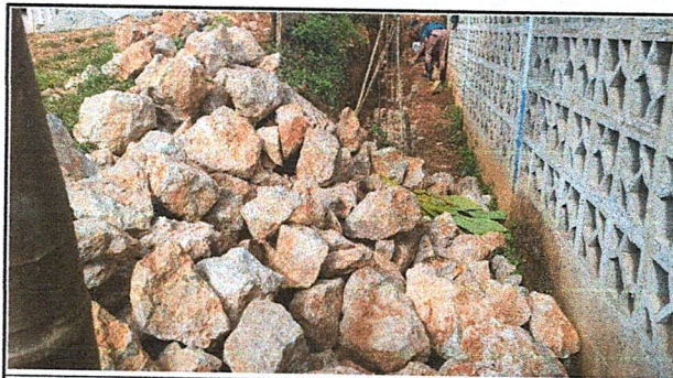
Foto 15: Reparación de muro de contención
