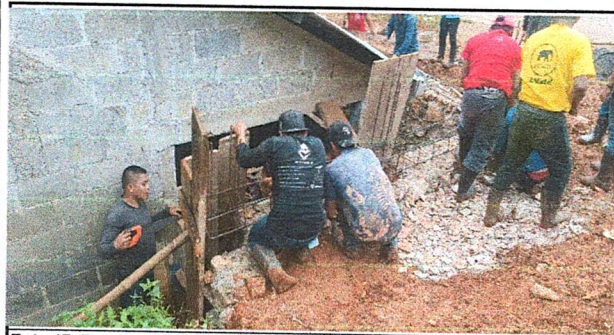
Foto 17. Reparación de muro de contención
